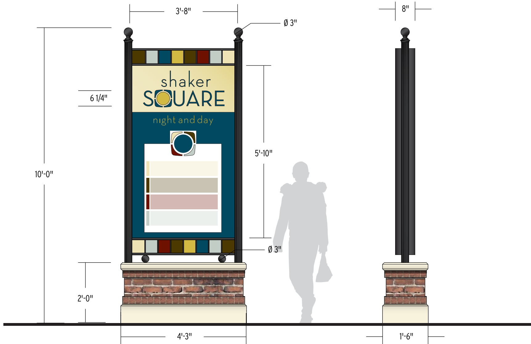
Option 2 - scale: 1/2" = 1'
